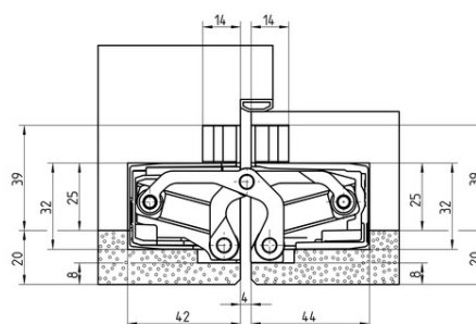
Dwarsdoorsnede 1
